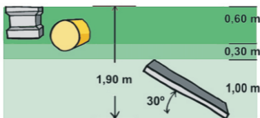
Alturas Mínimas com Reservatório de Nível
