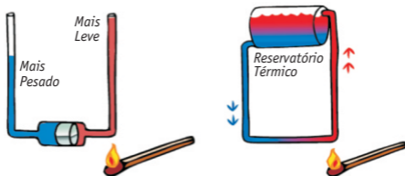
Exemplo de funcionamento por termossifão
