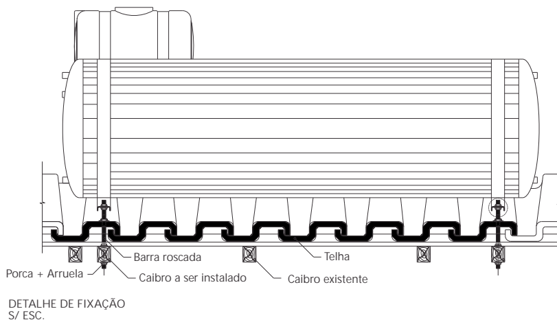
Vista dos detalhes de fixação do reservatório térmico sobre o telhado
